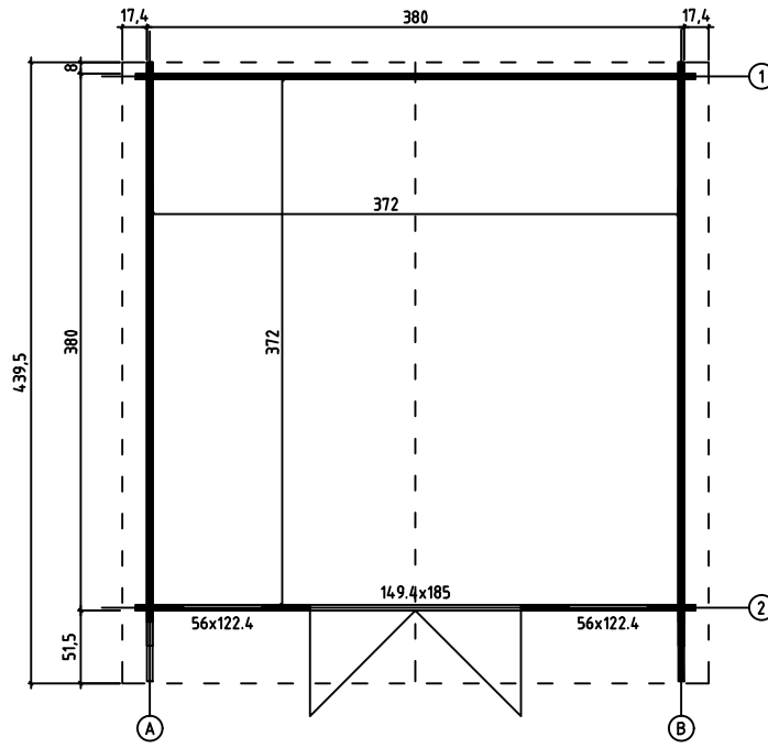
FOUNDATION - FUNDAMENT - FONDATION
