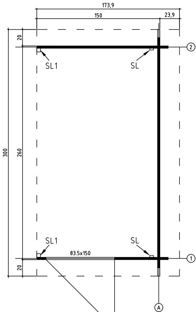
GROUNDPLAN - GRUNDPLAN - PLAN DE MASSE
