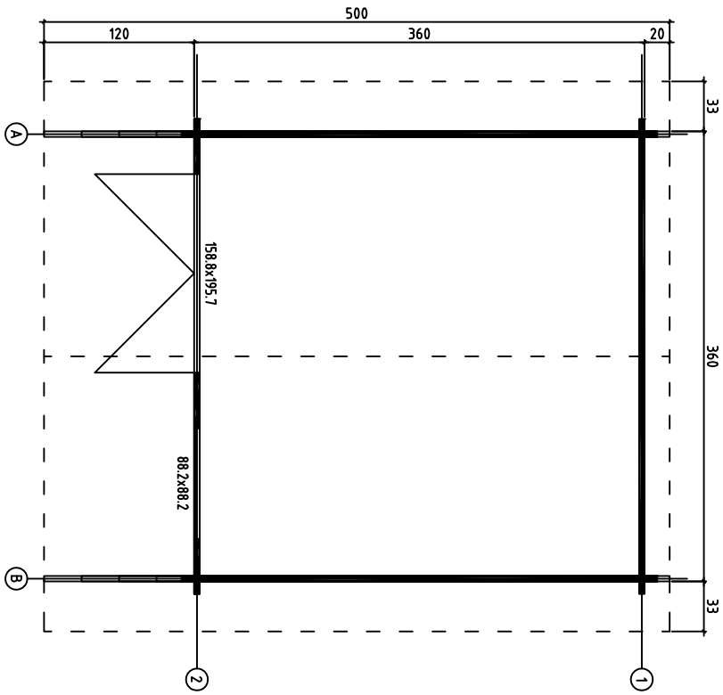
GROUNDPLAN - GRUNDPLAN - PLAN DE MASSE
